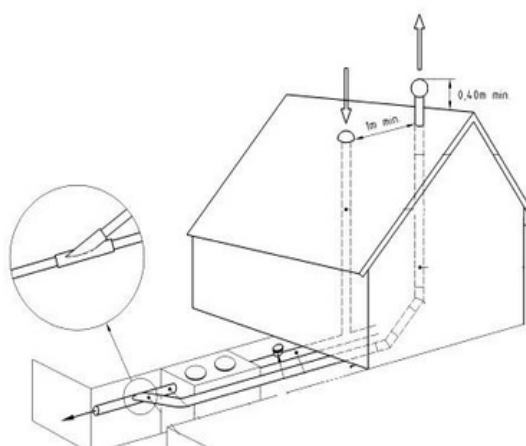
Figure 36 : raccordement des ventilations vers l'extérieur
