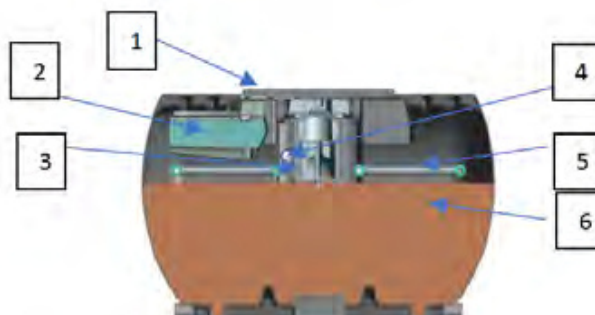
Figure 2 : Principaux composants du filtre compact
