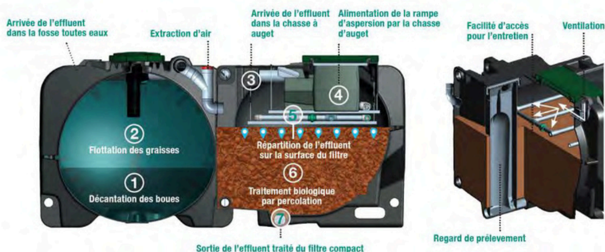
Figure 1 : Schéma de principe du pack BIONUT 2
