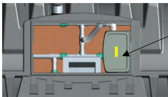
Figure 23 : Vue de dessus du filtre compact
