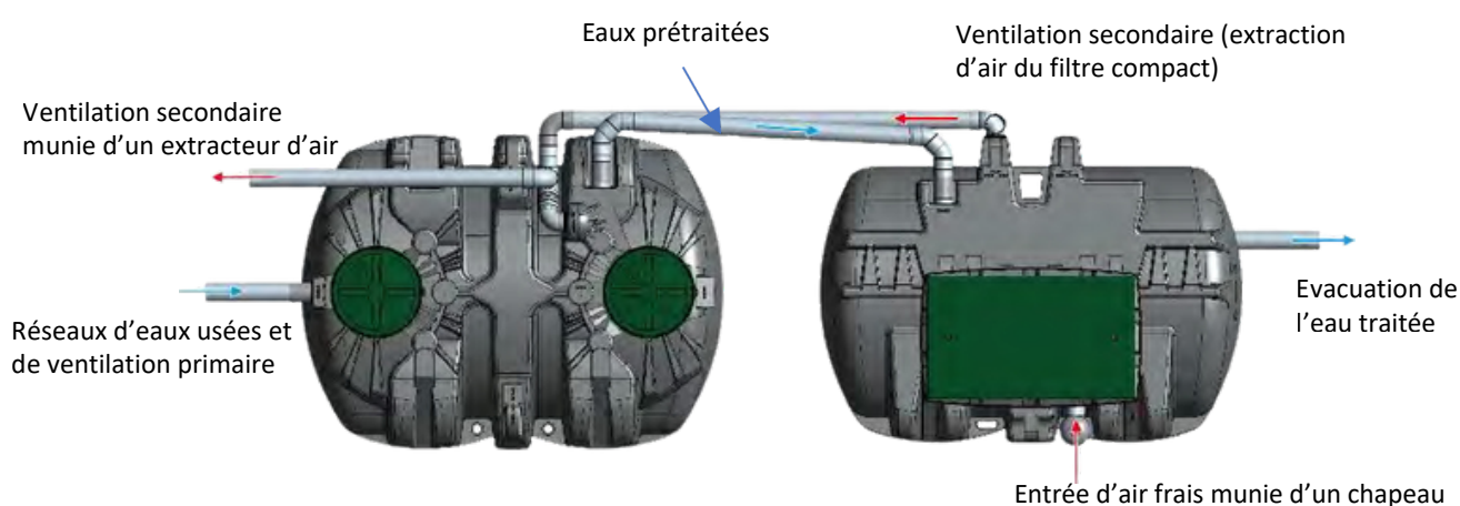
Figure 35 : ventilations primaires et secondaires (modèle 6 EH en ligne)
