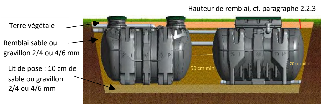
Figure 30 : Vue en coupe de l'installation en terrain normal, avec une pose en ligne
