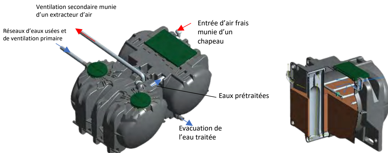
Figure 35 : ventilations primaires et secondaires (modèle 6 EH en pack)
