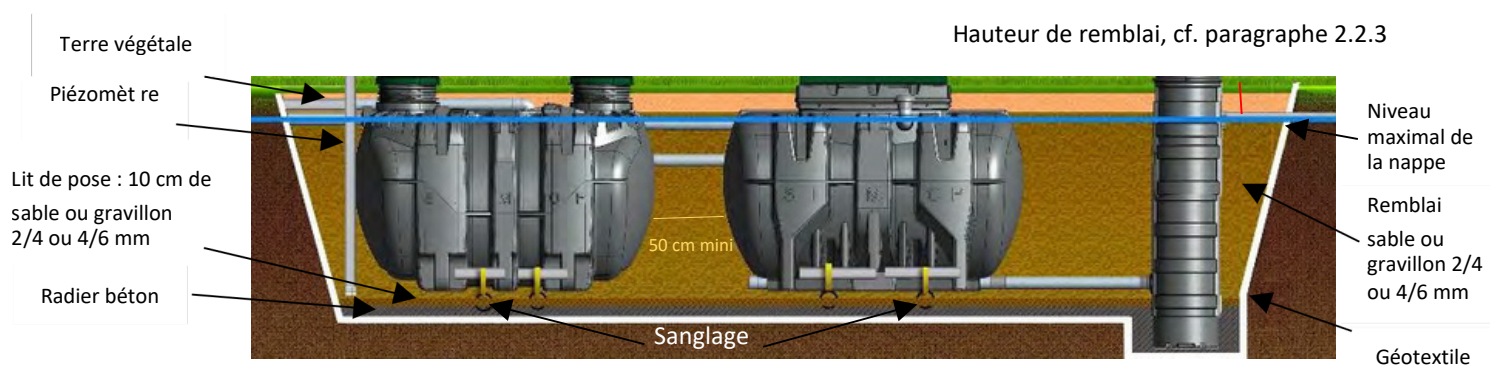
Figure 32 : schéma de pose en présence de nappe et/ou sol argileux
