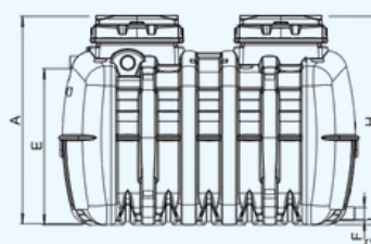
Vue latérale du filtre BIONUT2/08
