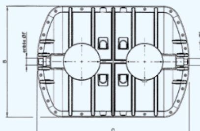
Vue de dessus de la FTE2/6309/10
