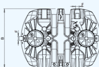
Vue de dessus de la FTE03000BI
