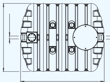
Vue de dessus de la INR06000 et INR08000
