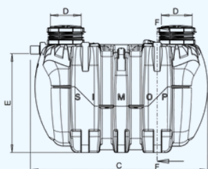
Vue latérale de la FTE03000BI
