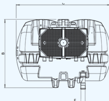
Vue de dessus du filtre BIONUT2/04 à 06
