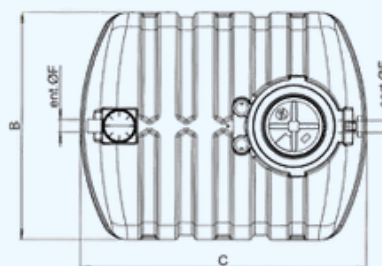
Vue de dessus de la FTE2/6009/04 (pour BIONUT2/6054/08)
