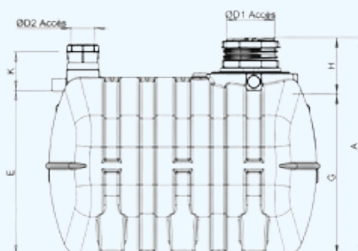
Vue latérale de la FTE2/6009/04 (pour BIONUT2/6054/08)
