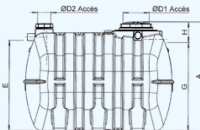
Vue latérale de la FTE2/6009/05 (pour BIONUT2/6054/10)
