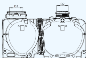
Vue de face du pack BIONUT2/6054/04 à 06
