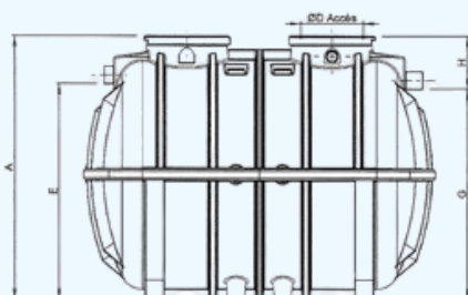
Vue latérale de la FTE2/6309/10
