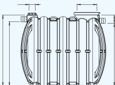
Vue latérale de la INR06000 et INR08000
