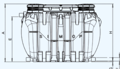
Vue latérale du pack BIONUT2/6054/04 à 06
